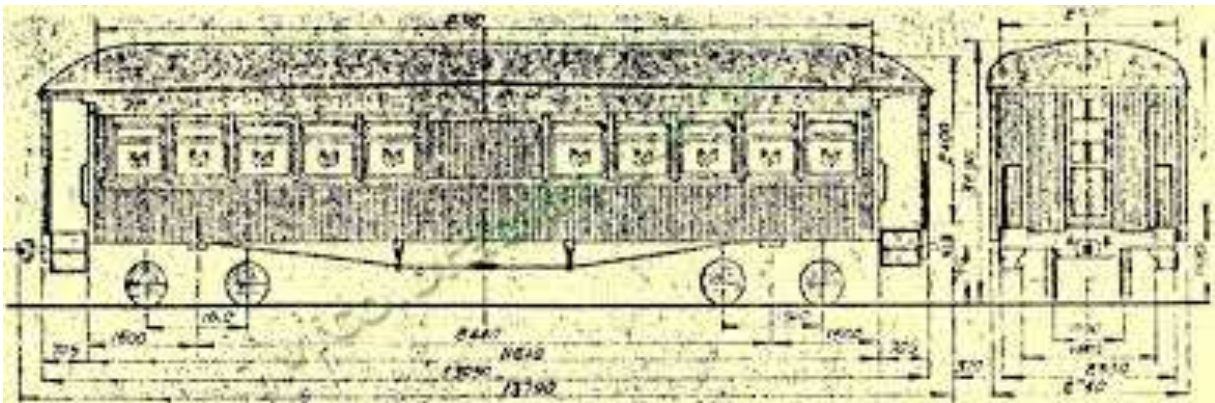
Projeto Original do Vagão de Madeira – Passageiros Modelo carro de passageiros de Primeira Classe nº 115
